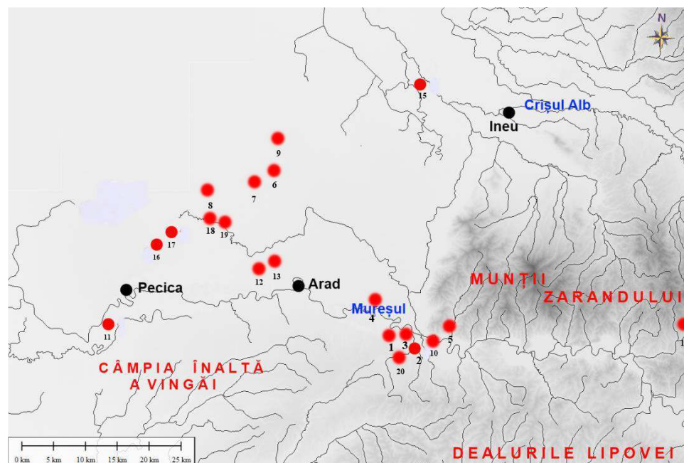
Fig.1. Localizarea structurilor de pământ din județul Arad descoperite pe imaginile satelitare Google Earth (2014-2017).
