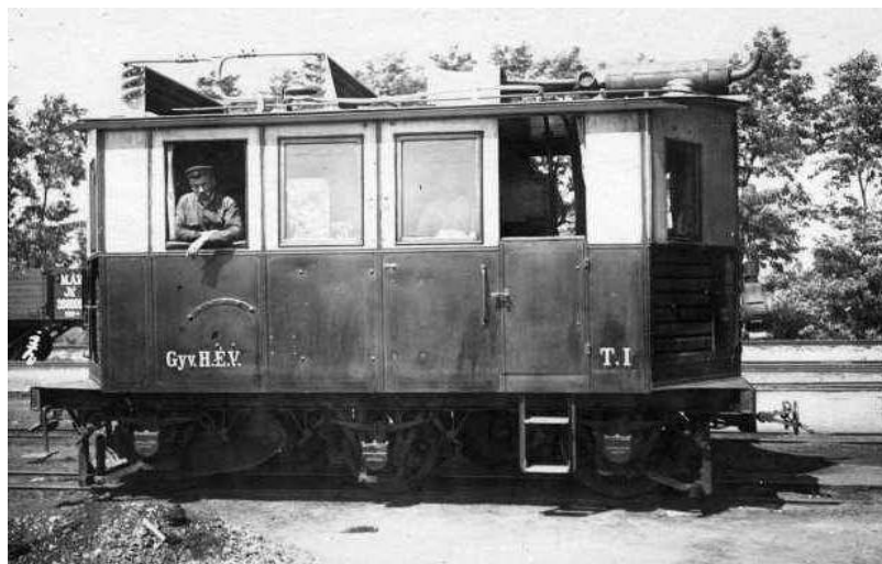
Automotor benzo electric produs la fabrica Johann Weitzer din Arad
