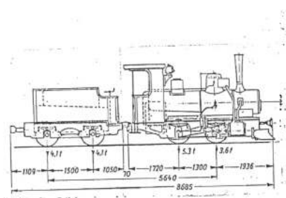
Locomotiva tip Bn2 seria MAV 288, categoria XXib, constructor J. Weltzer - Arad, 1898
