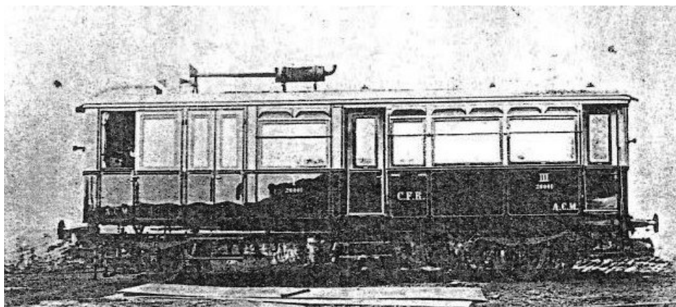
Foto : Automotor cu ecartament de 760mm produs de fabrica Johann Weitzer din Arad cu motorizare De Dion-Bouton
