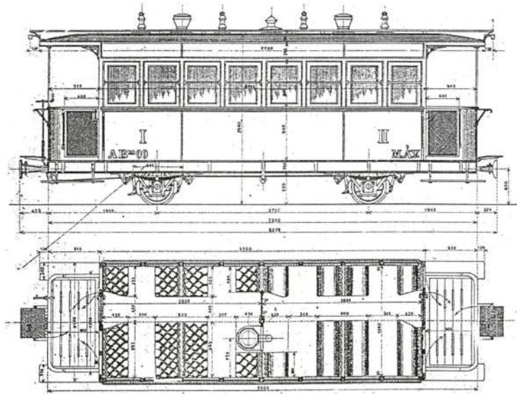
Foto Plansa vagon de calatori ci. I ( numar de locuri 11) si cl .III ( numar de locuri 11) produs la fabrica Johann Weitzer din Arad incepind cu anul 1985, a fost utilizat de MAV si de liniile HEV Gyulavidek respectiv Alba Iulia –Zlatna.
