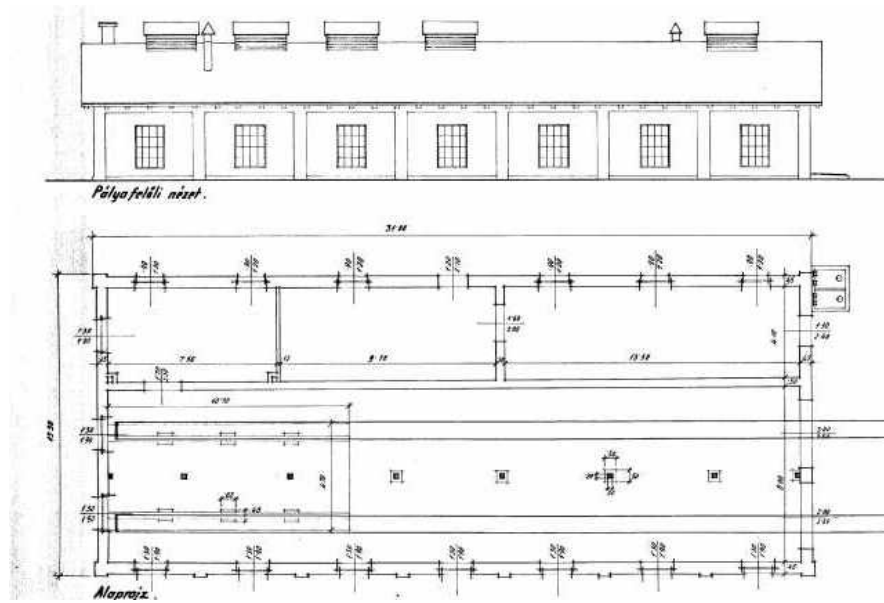
Schita halei depoului HEV Gyulavidek
