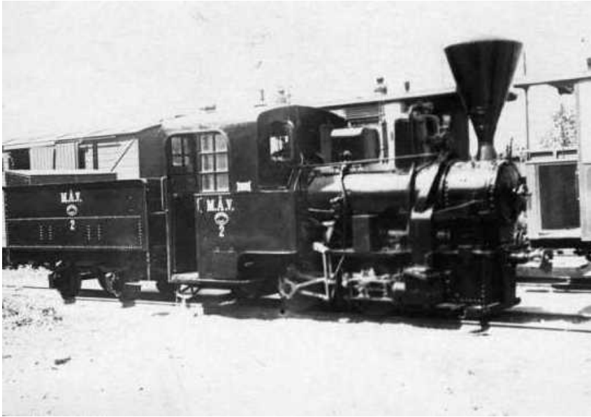
Locomotiva tip produsa la fabrica Johann Weitzer din Arad este inregistrata de catre M.A.V. in anul
