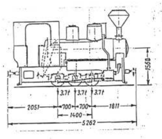
Locomotiva tip Ctn2 seria MAV 399, constructor Budapesta 1906 - 1913
